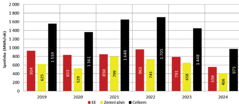
Vývoj reálných spotřeb energií za 2019–2024 Porovnání prostých spotřeb energií Nový Malín
